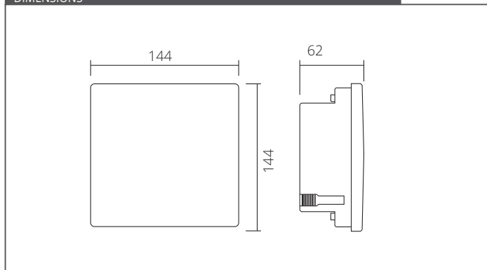
DIMENSIONS
